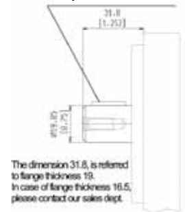
Key 4,78x4,78x12,7
