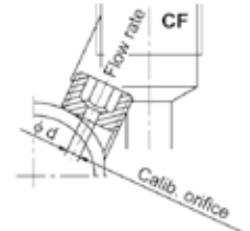
Det. SECTA-A
